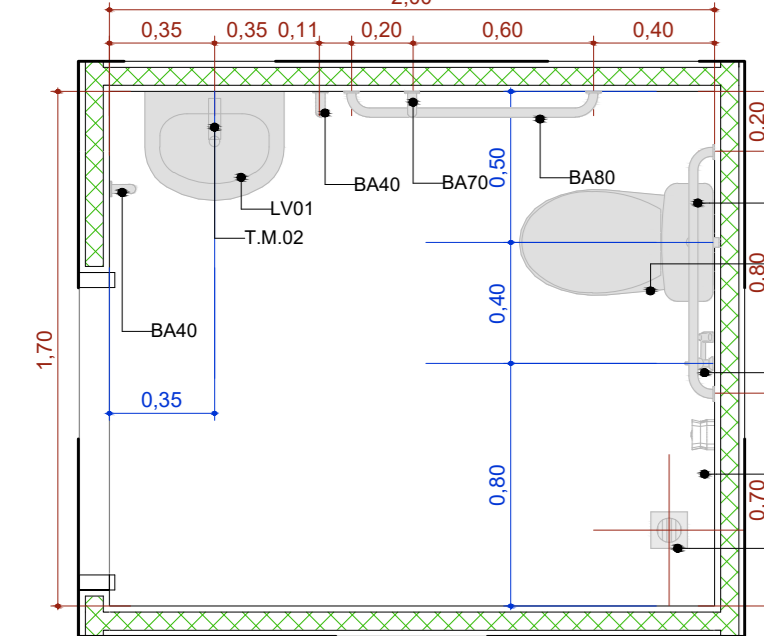
A.M.3 Sanitário PCD Masc. Escala: 1:25
