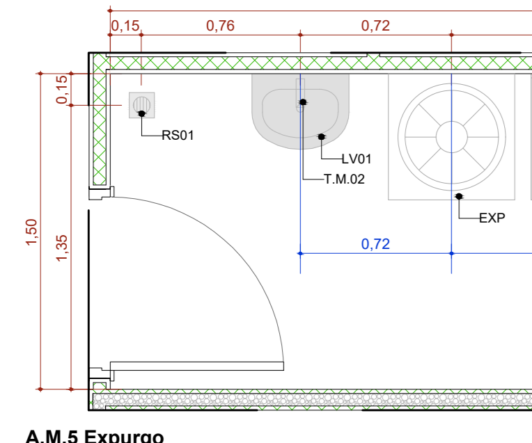
A.M.5 Expurgo Escala: 1:25
