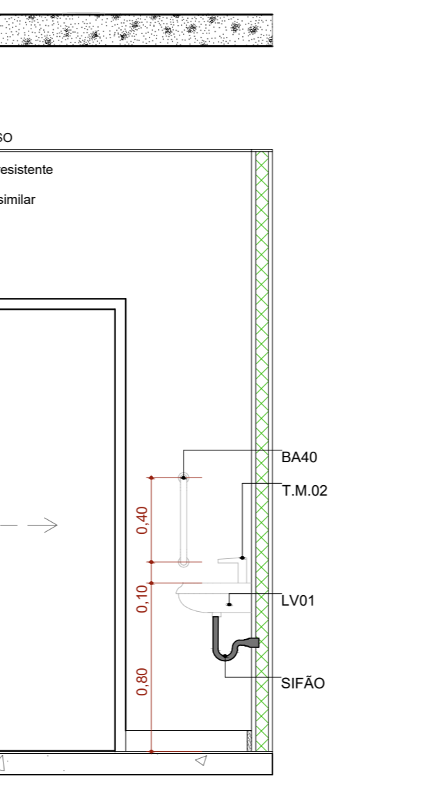
A.M.04 VISTA 1 Escala: 1:25
