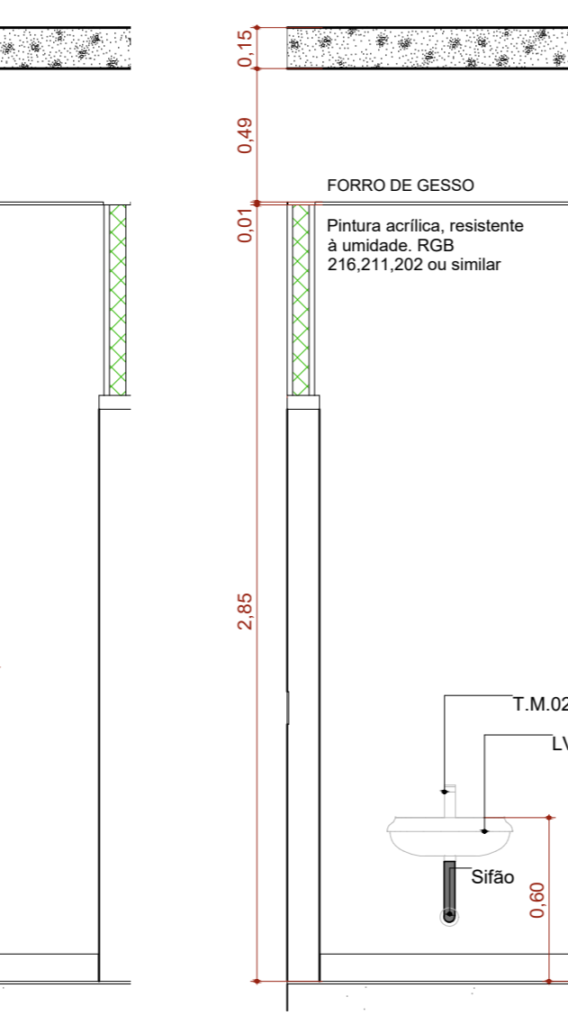
A.M.01 VISTA 4 Escala: 1:25
