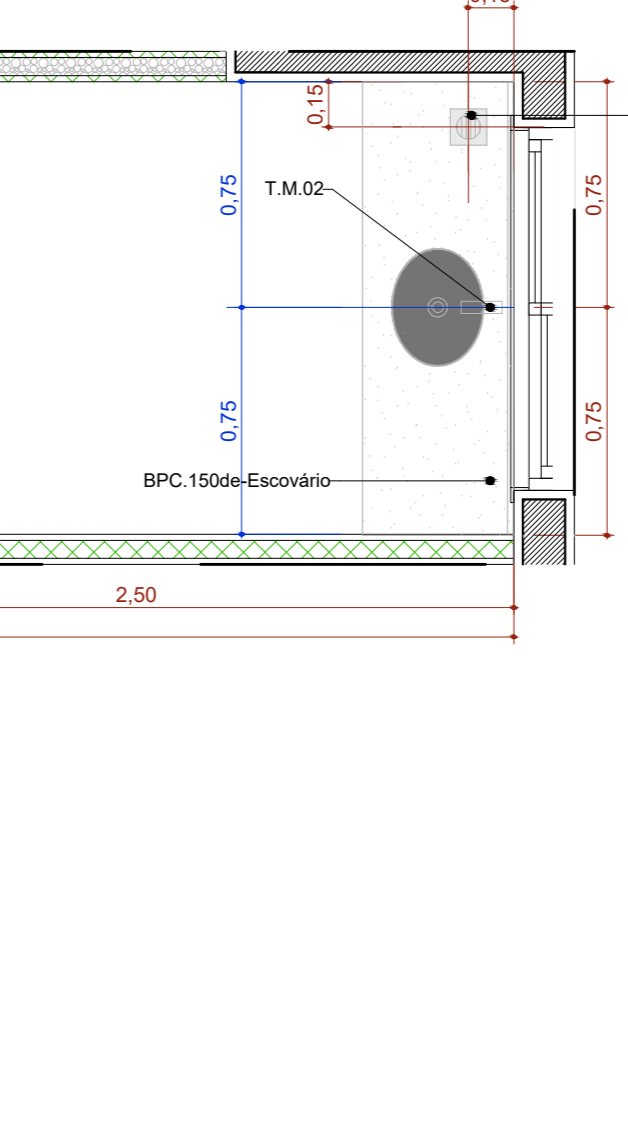
A.M.04 VISTA 3 Escala: 1:25
