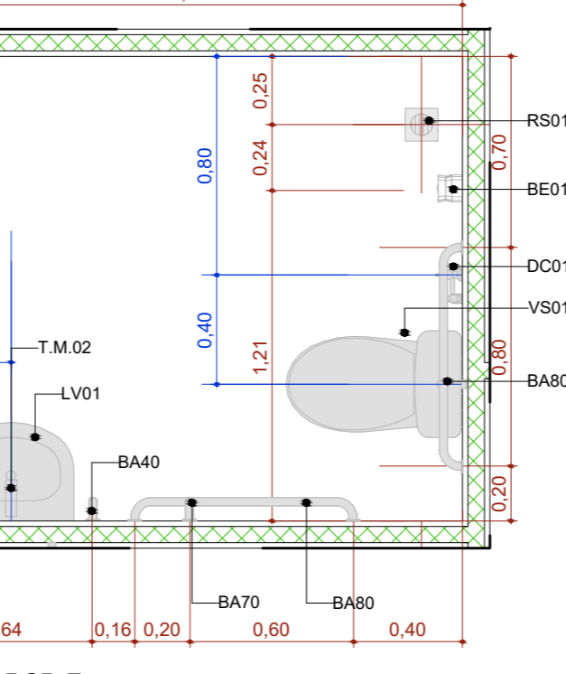
A.M.2 Sanitário PCD Fem. Escala: 1:25
