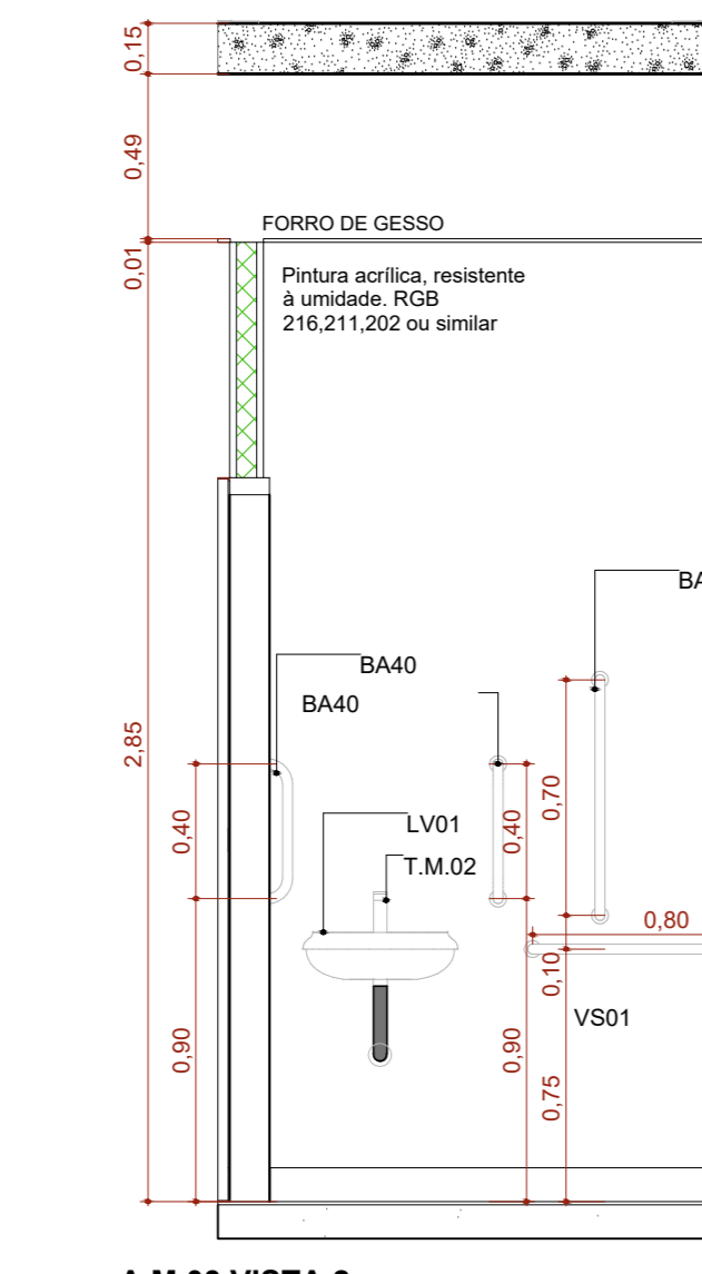
A.M.03 VISTA 2 Escala: 1:25
