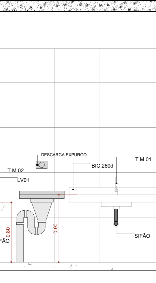
A.M.05 VISTA 3 Escala: 1:25
