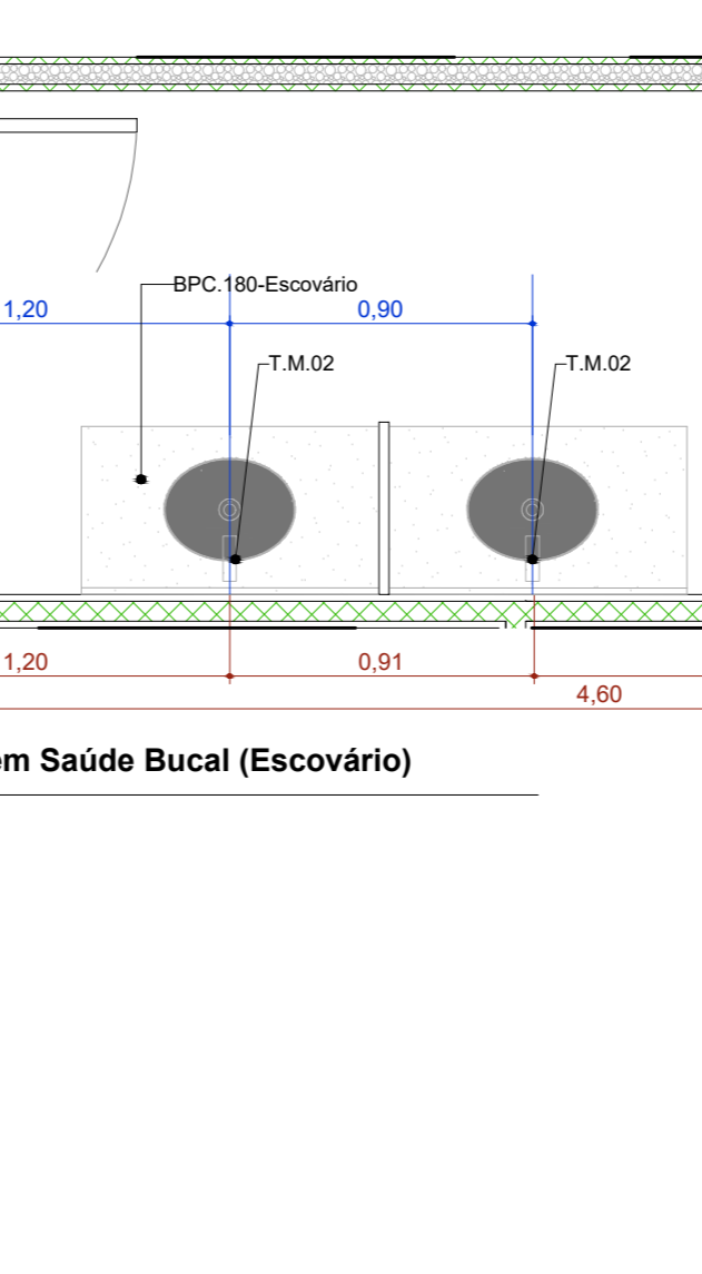
A.M.04 VISTA 2 Escala: 1:25
