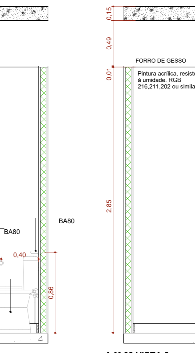
A.M.03 VISTA 3 Escala: 1:25
