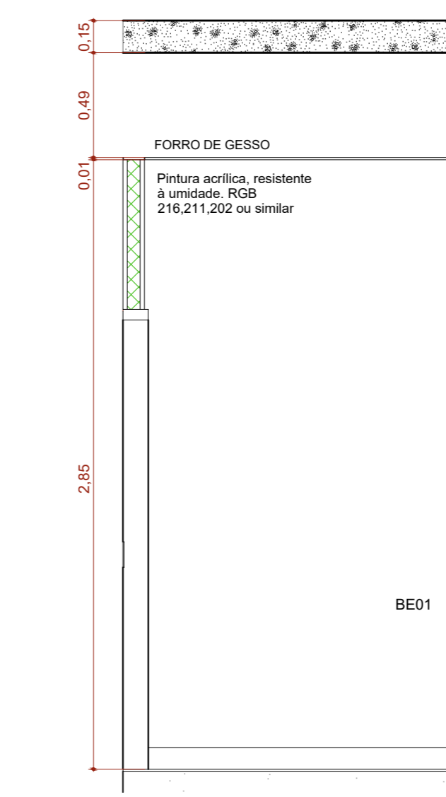
A.M.02 VISTA 2 Escala: 1:25
