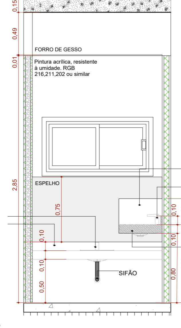
A.M.06 VISTA 3 Escala: 1:25
