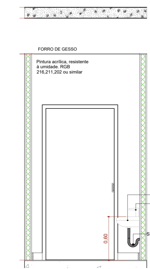
A.M.01 VISTA 2 Escala: 1:25
