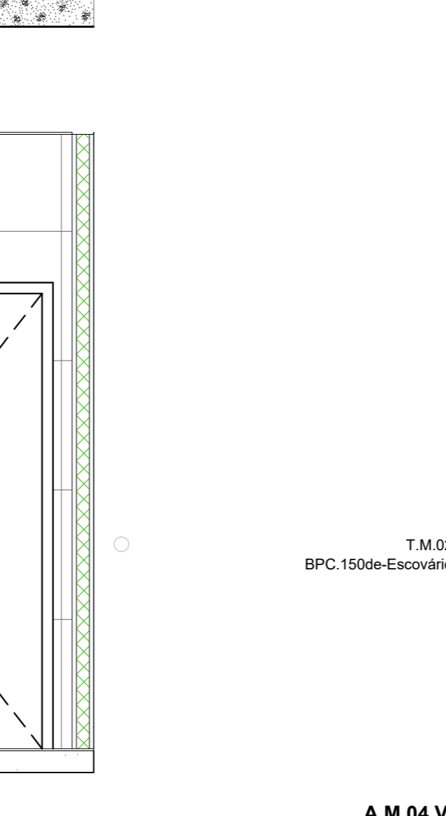
A.M.06 VISTA 2 Escala: 1:25
