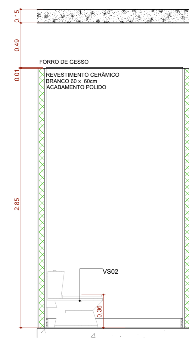
A.M.01 VISTA 1 Escala: 1:25
