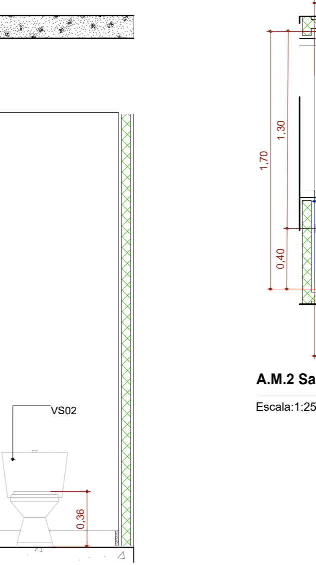
A.M.02 VISTA 1 Escala: 1:25
