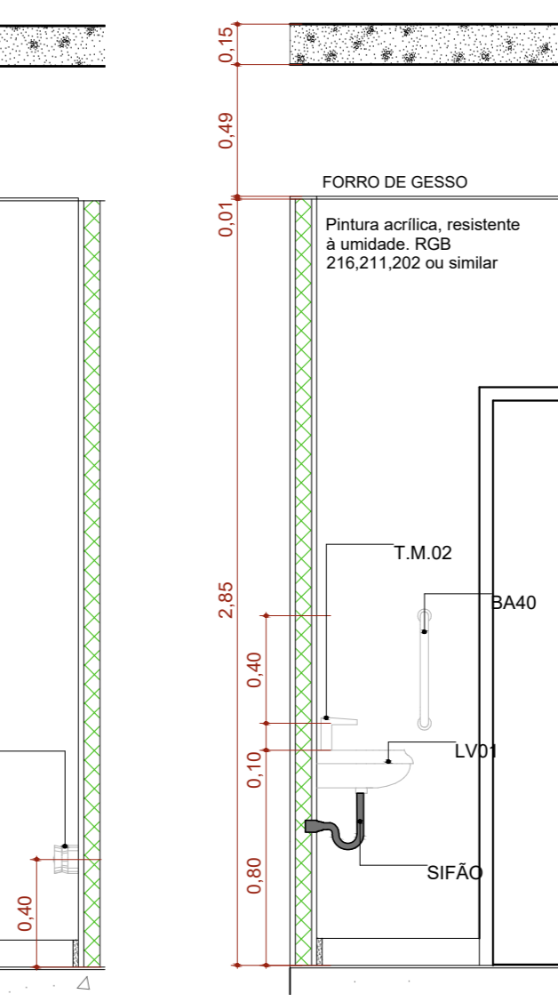
A.M.02 VISTA 3 Escala: 1:25
