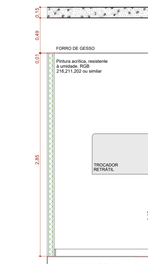
A.M.01 VISTA 3 Escala: 1:25
