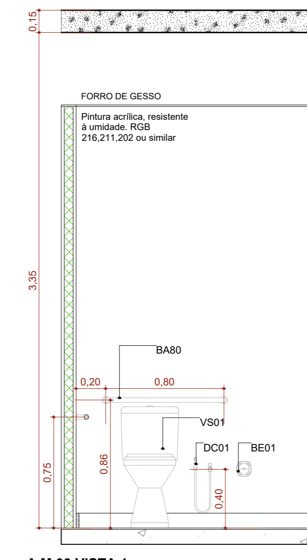
A.M.03 VISTA 1 Escala: 1:25
