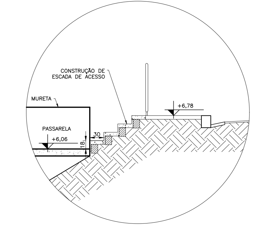
CORTE C-C - CONSTRUÇÃO Esc. 1:50
