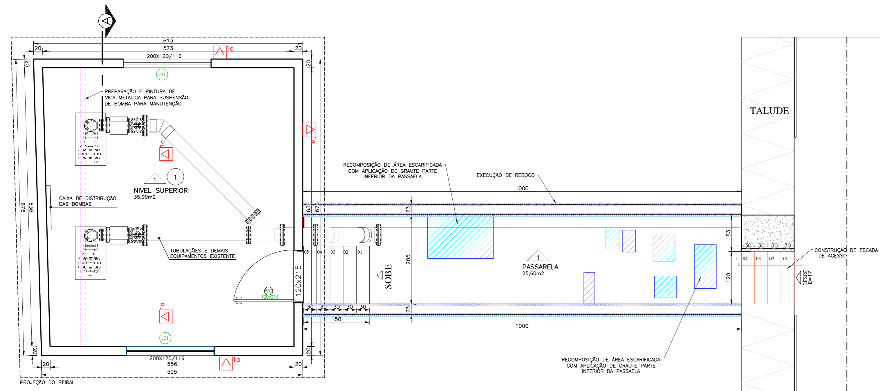
PLANTA DE CONSTRUÇÃO - NÍVEL SUPERIOR Esc. 1:50
